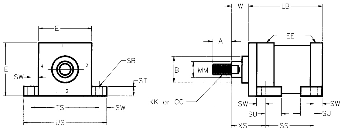
MS2 SIDE LUG
