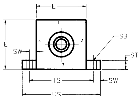
MS2 SIDE LUG
